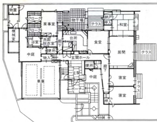
1 階平面図
