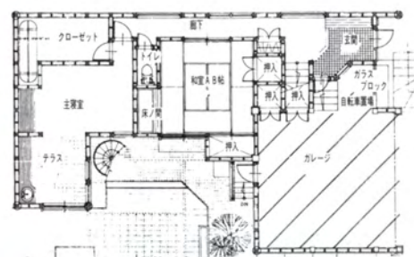
1階平面図
