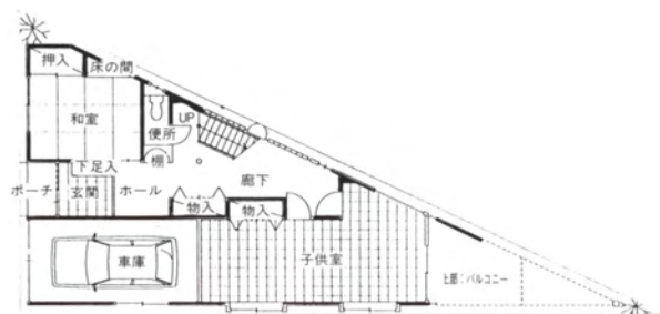
1階平面図
