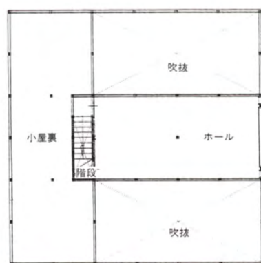
3階平面図
