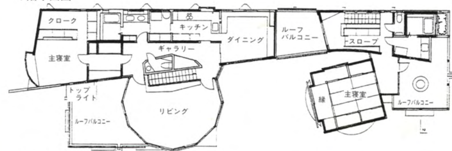
2階平面図
