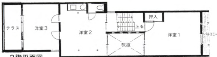
2階平面図
