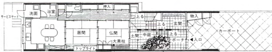
1 階平面図
