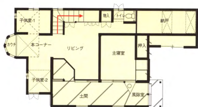
1 階平面図
