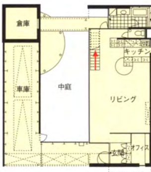
1 階平面図
