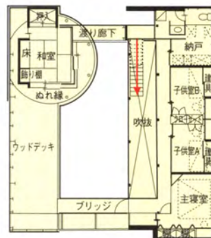
2 階平面図
