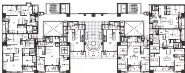
8階平面図
