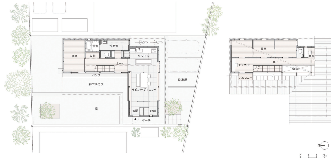
配置・平面図
